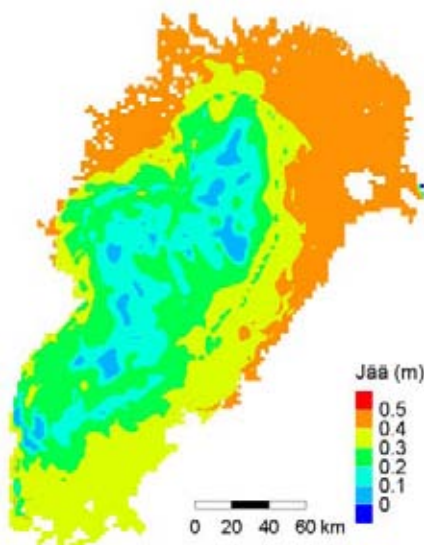
Laskettu jäättilanne 27.01.2003 12:00
