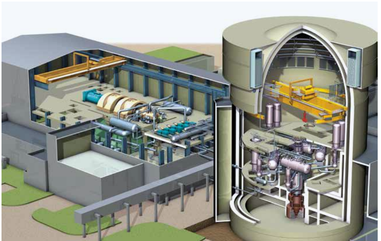
AES-2006-laitoksen poikkileikkaus.
